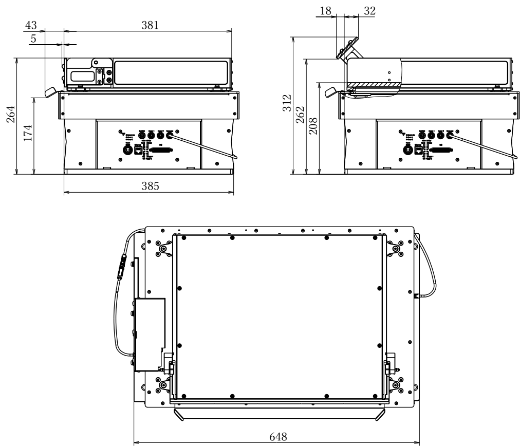
IF-A3540 (排出扉/右)
