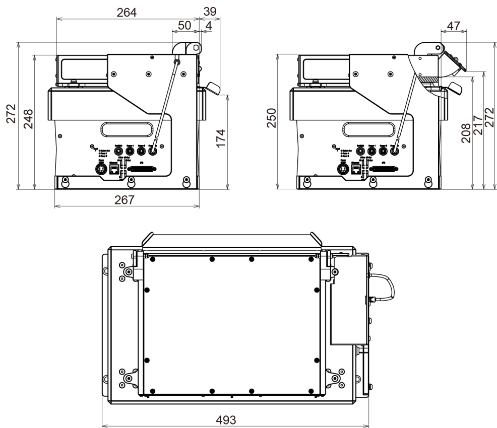
IF-A3540 (排出扉/左)
