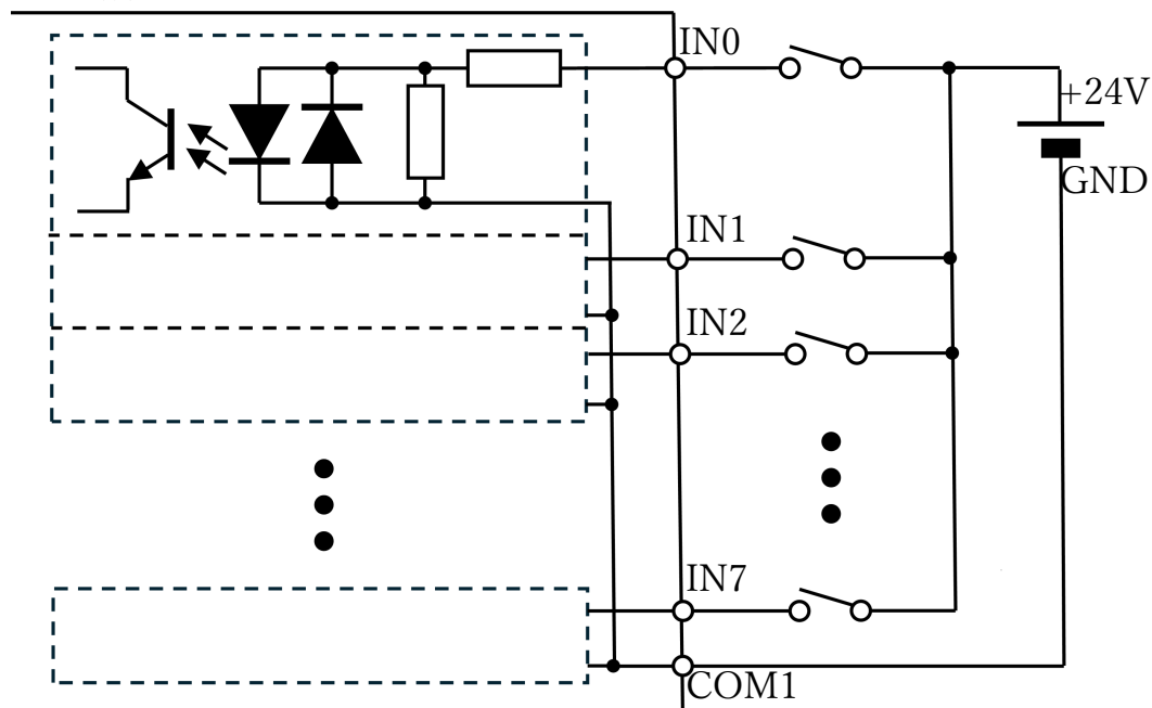
入力配線例1
