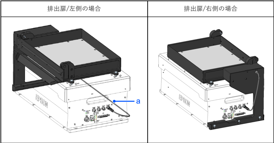
参考:取り付け後のイメージ
