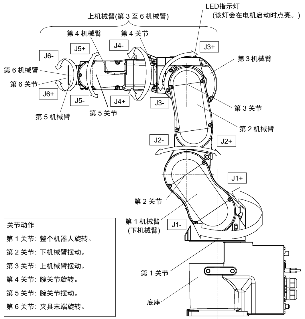
(图: C8-A701*(C8))
