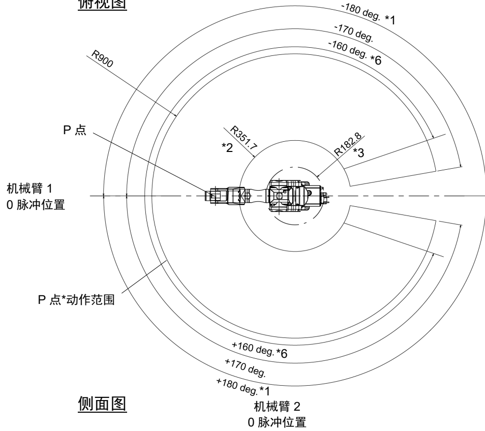
俯视图
