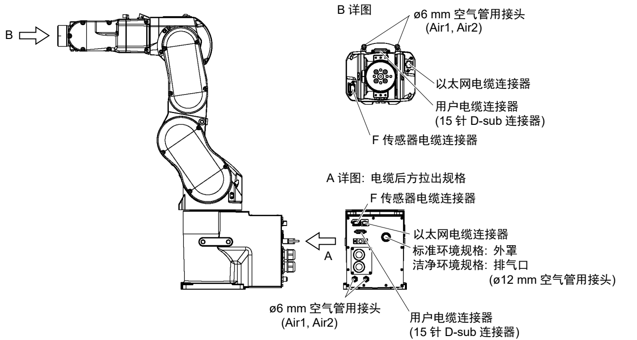
(图: C8-A701*(C8))
