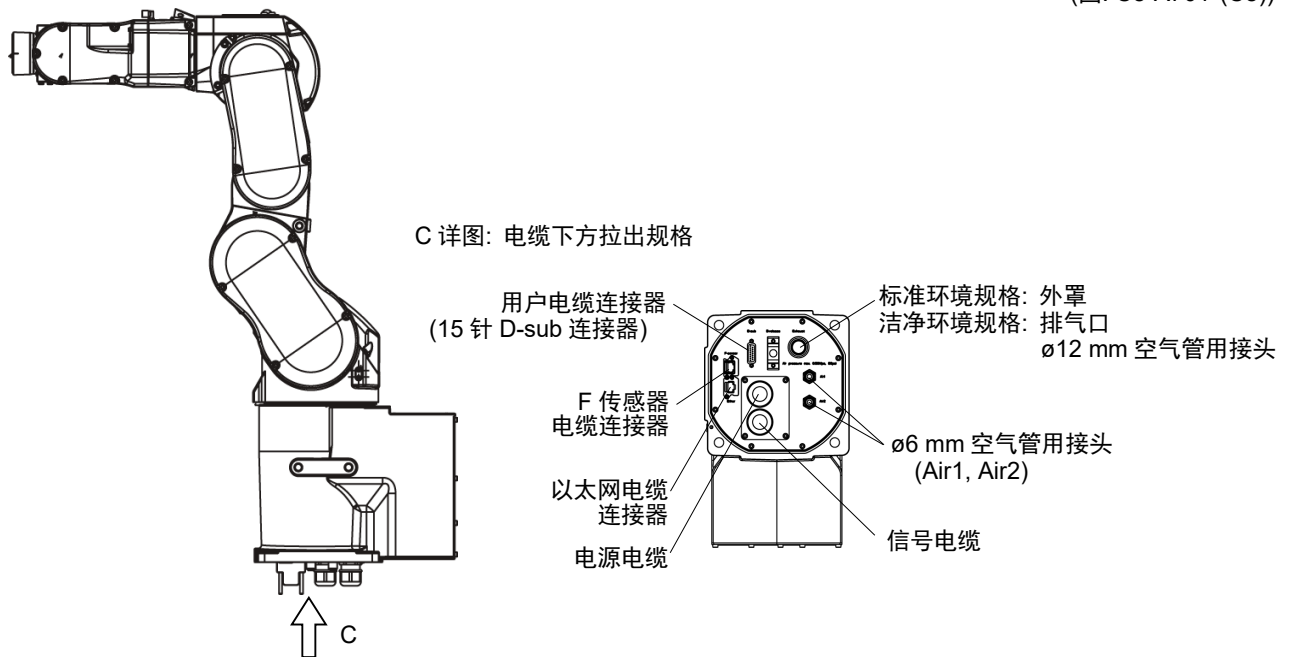
(图: C8-A701*B(C8))
