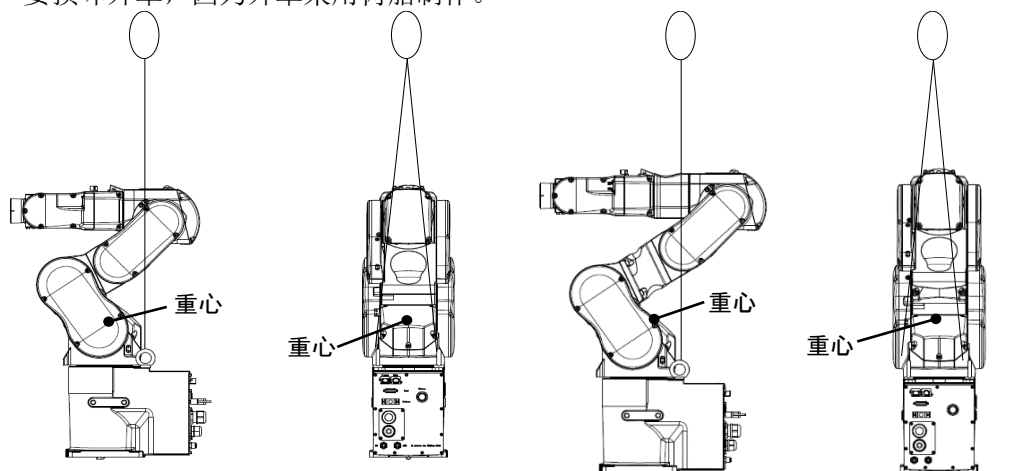
(图: C8-A701* (C8))
