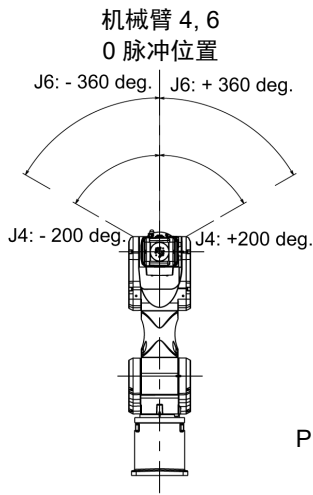
正面图
