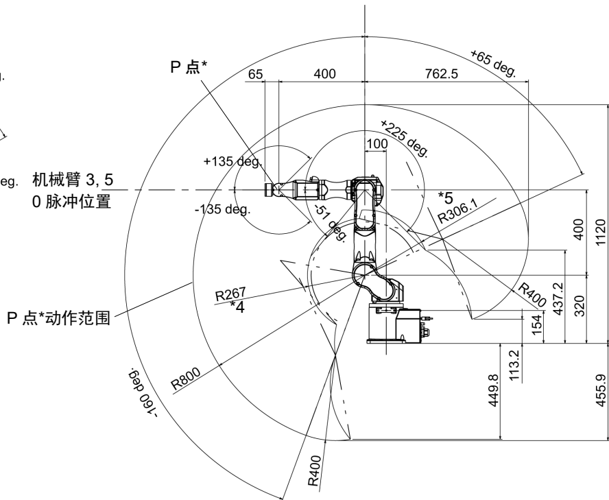
侧面图
