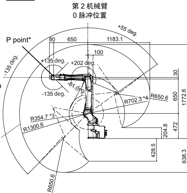
侧视图
