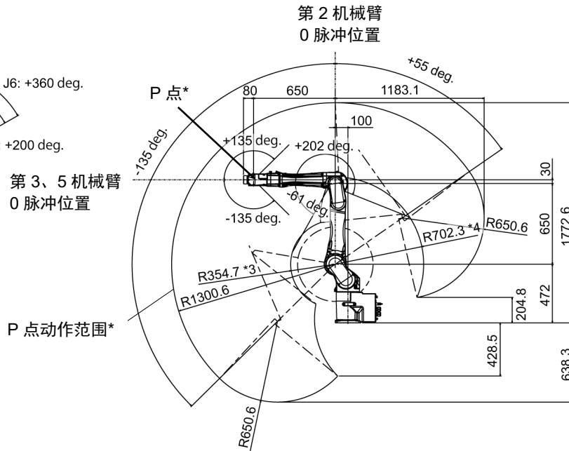
侧视图
