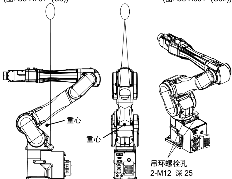
(图: C8-A1401*(C8XL))
