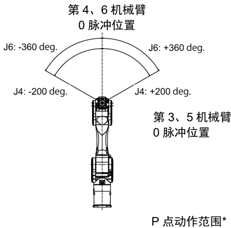
前视图
