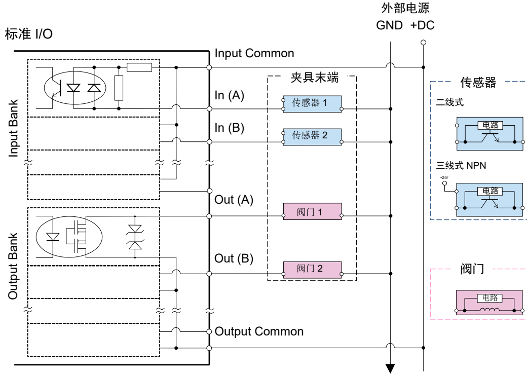
电路图示例(a)输入：正公共端子(法)、输出：正公共端子(法)
