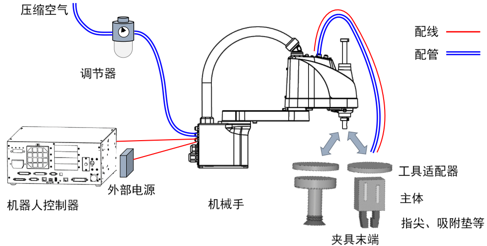
夹具末端安装概要图
