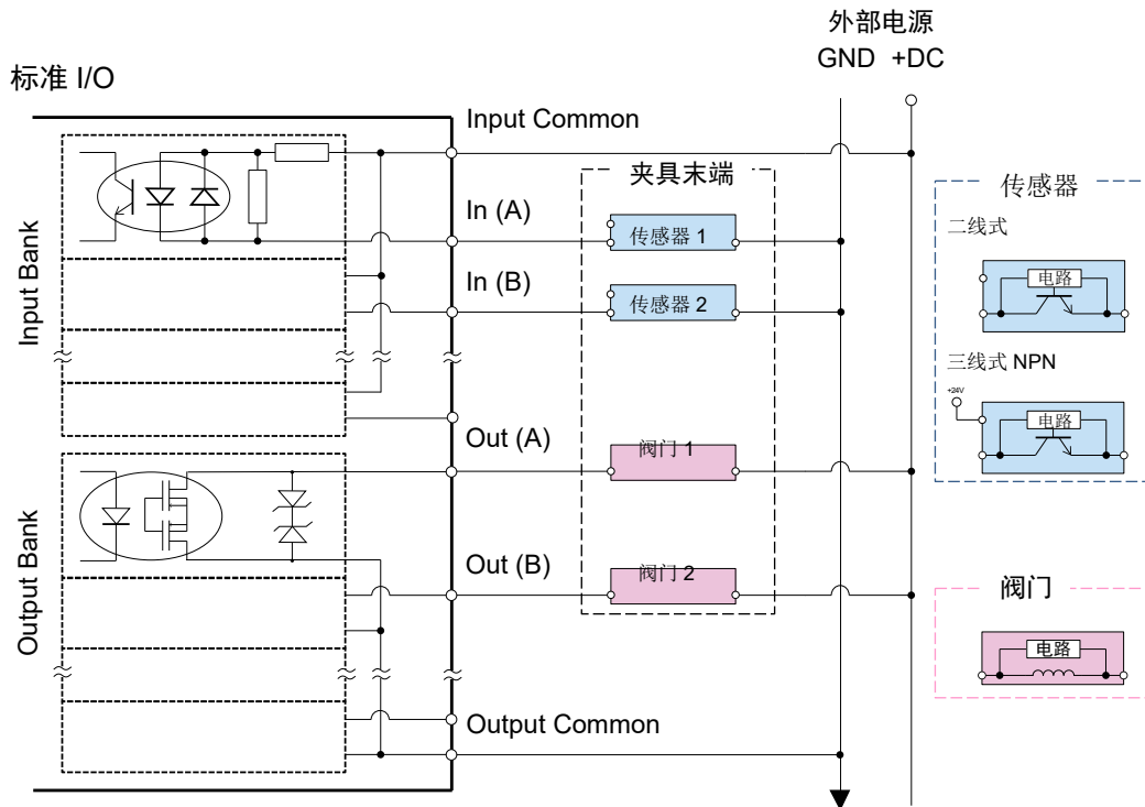
电路图示例(b)输入：正公共端子(法)、输出：负公共端子(法)
