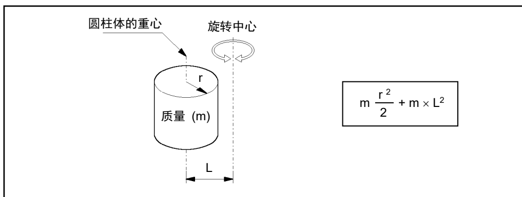
(b) 圆柱体的惯性力矩(Inertia)
