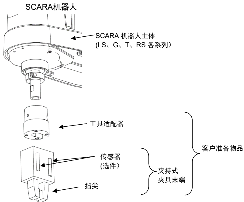
夹持式夹具末端安装概要图
