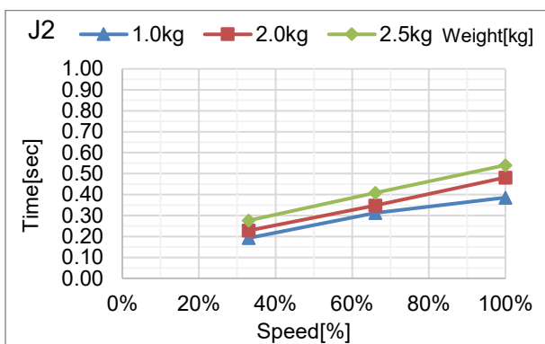
N2-A450S*: J2 (台面安装, 吊顶安装)
