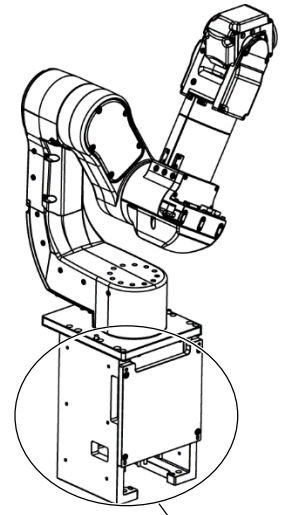
台面安装架
