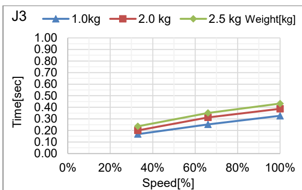
N2-A450S*: J3 (台面安装, 吊顶安装)
