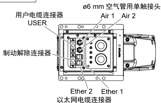
A 详图
