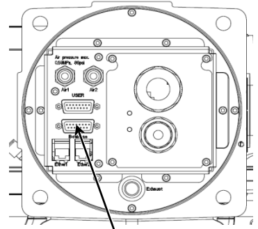
连接电缆连接器
