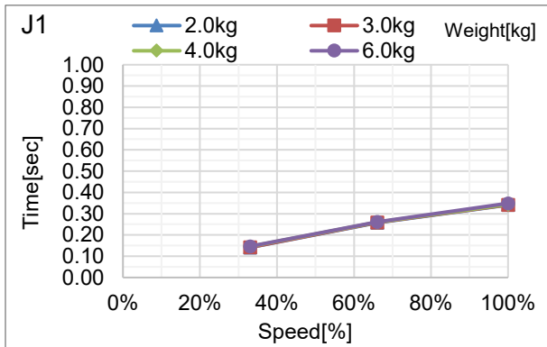
N6-A850**R: J1 (吊顶安装)
