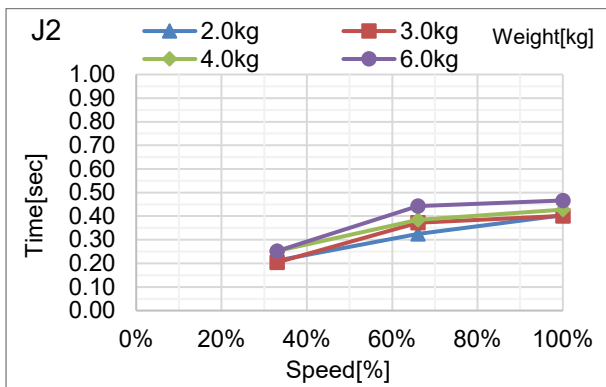
N6-A850**R: J2 (吊顶安装)
