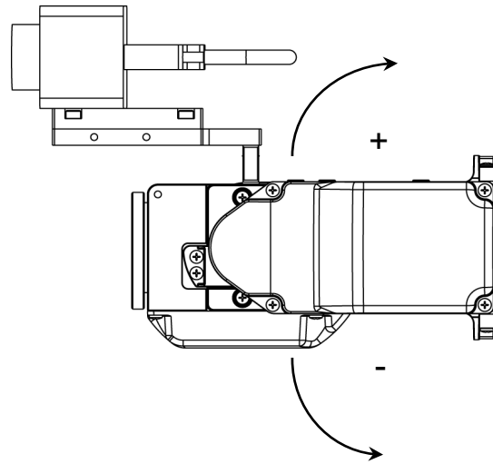
第5关节的动作方向
