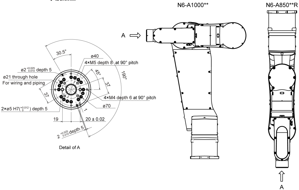
手腕法兰
