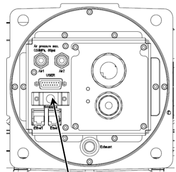
外部短接连接器
