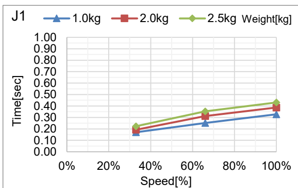
N2-A450S*: J1 (台面安装, 吊顶安装)
