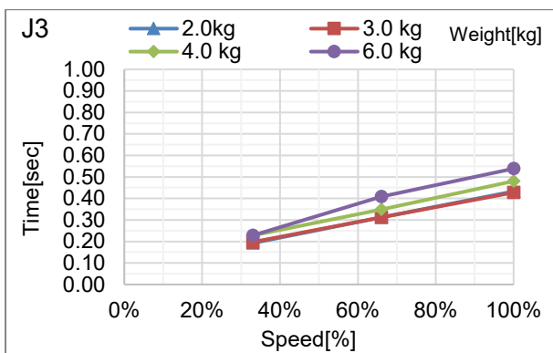
N6-A850**R: J3 (吊顶安装)
