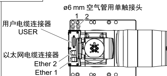
B 详图
