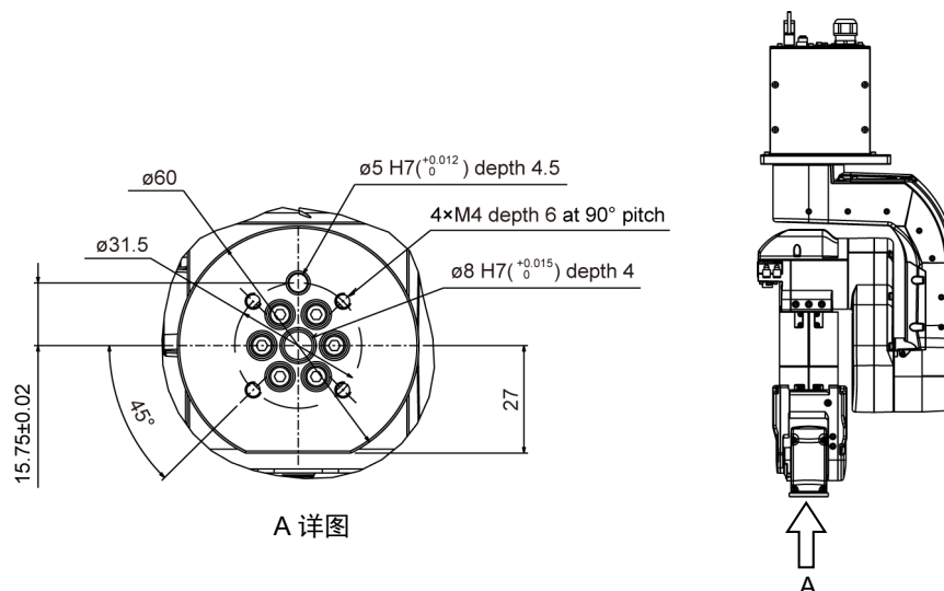
腕关节法兰
