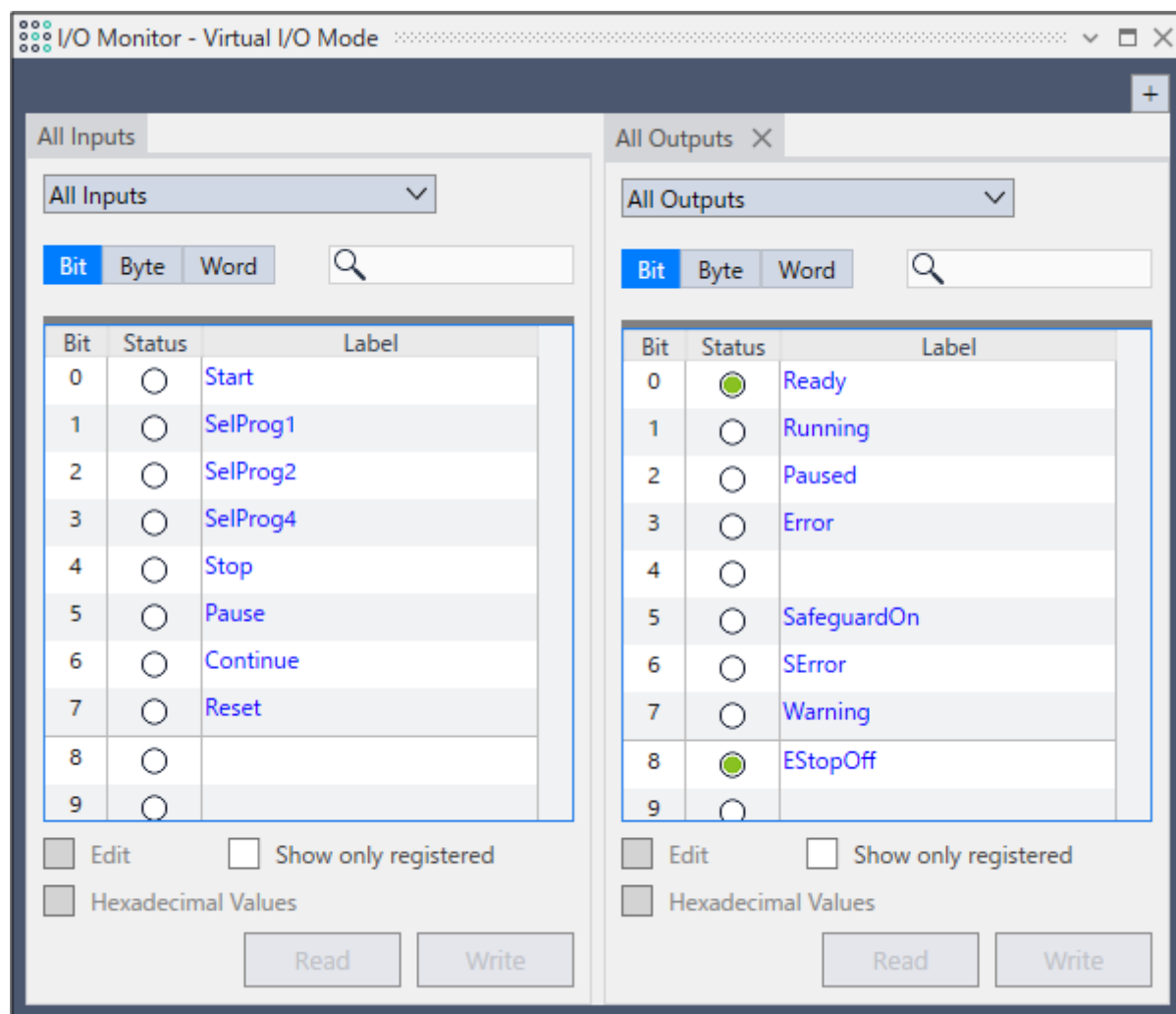
I/O Monitor 窗口
