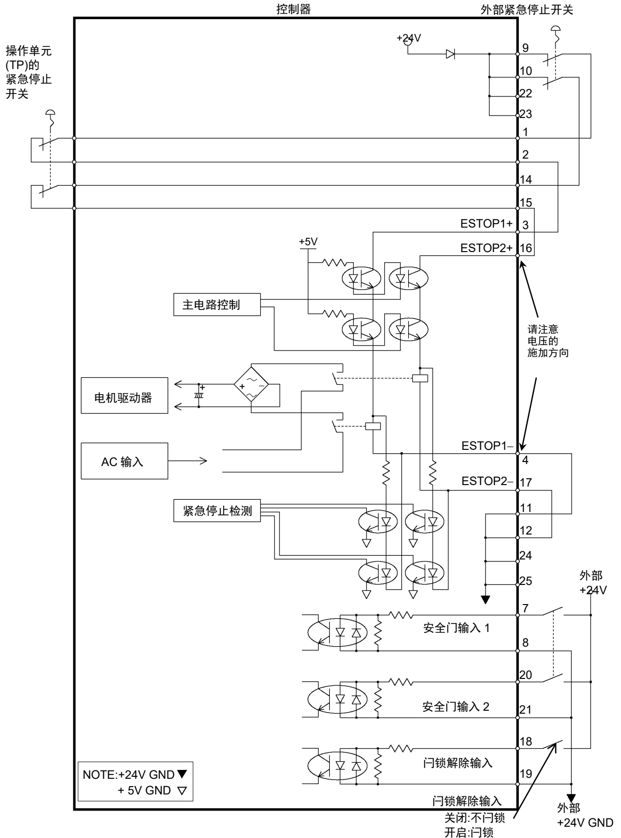
例 1：连接外部紧急停止开关时
