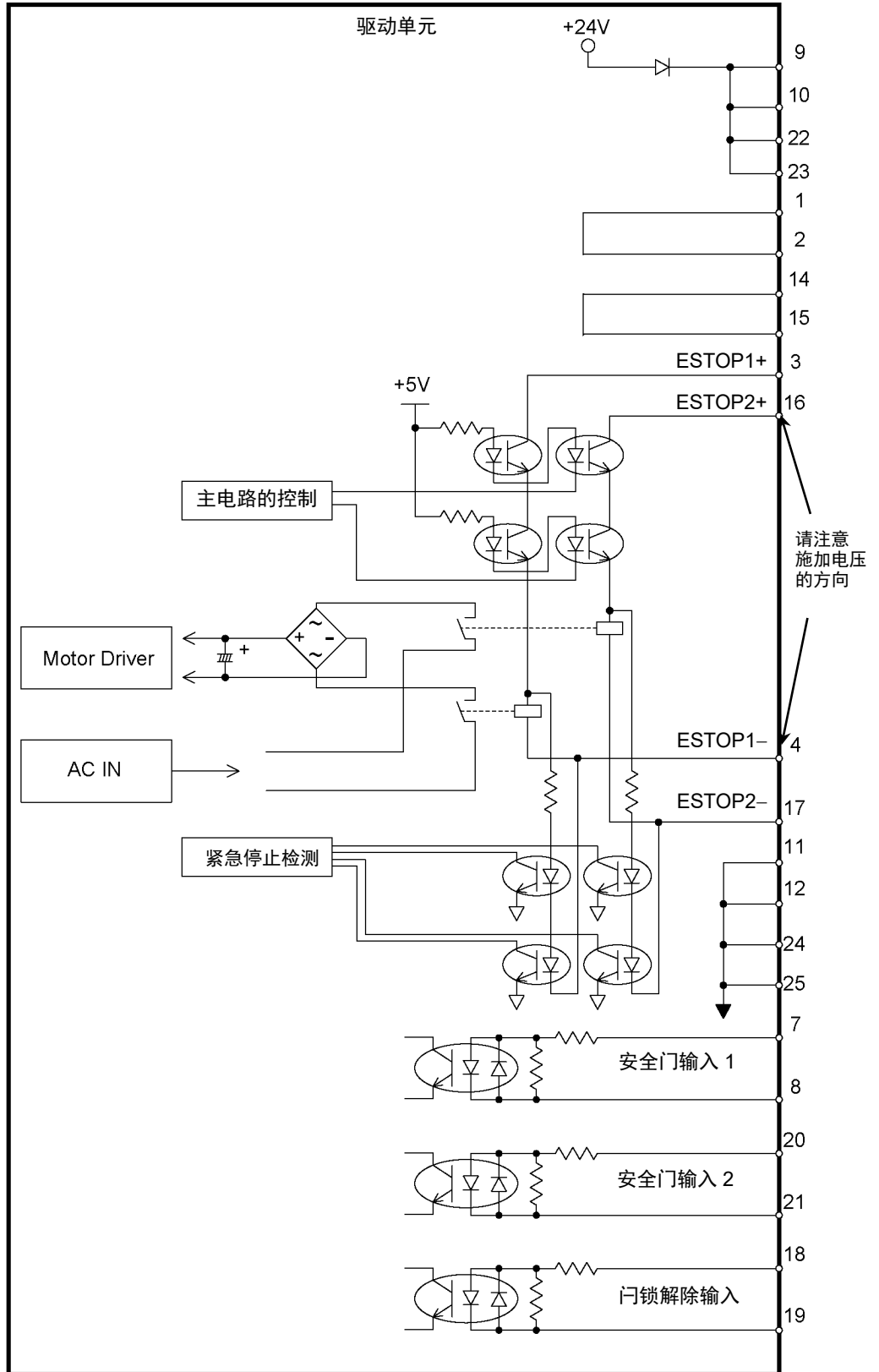
电路图
