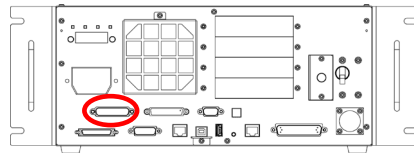
EMERGENCY 接头(图: RC700)
