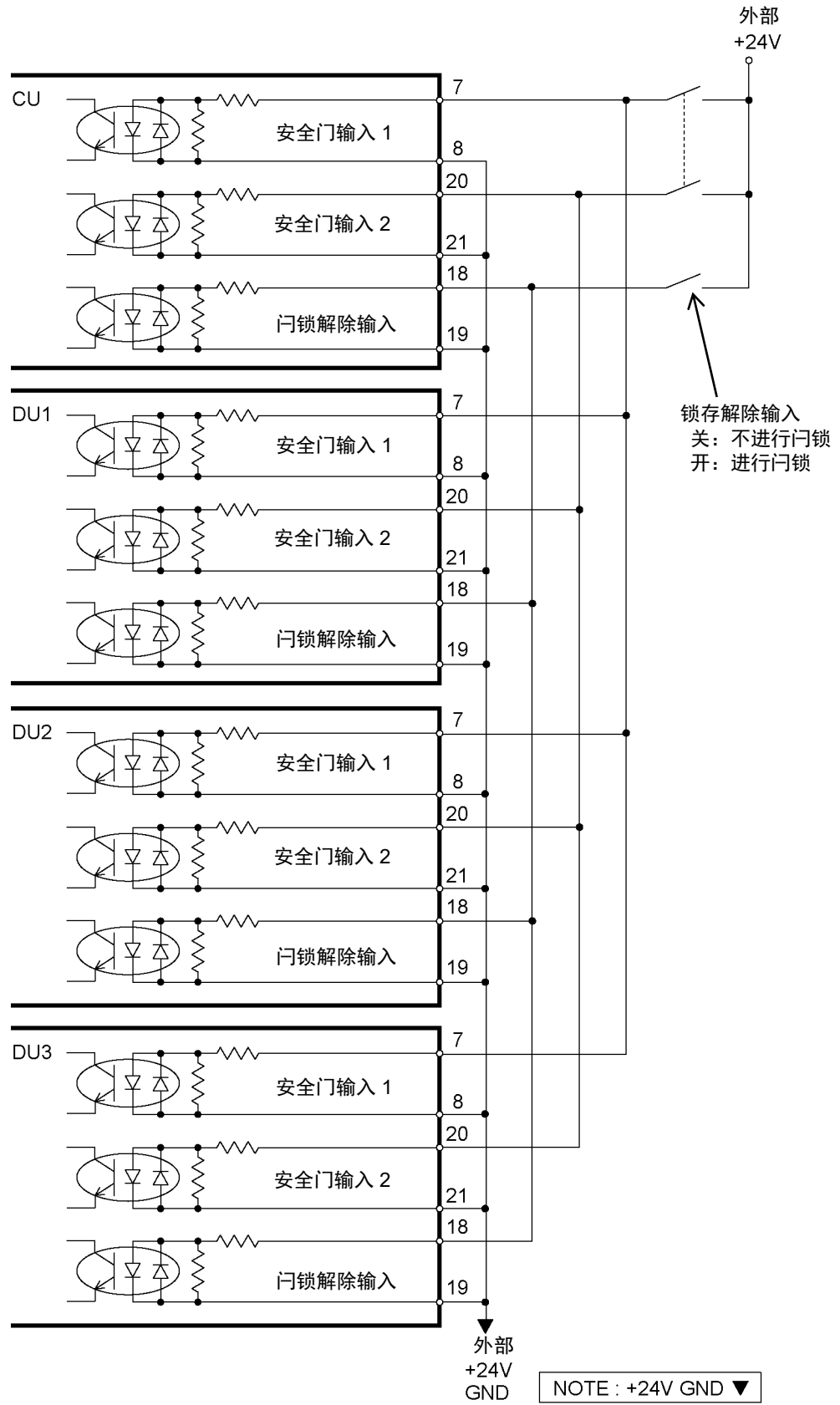
安全门输入与门锁解除输入的配线示例
