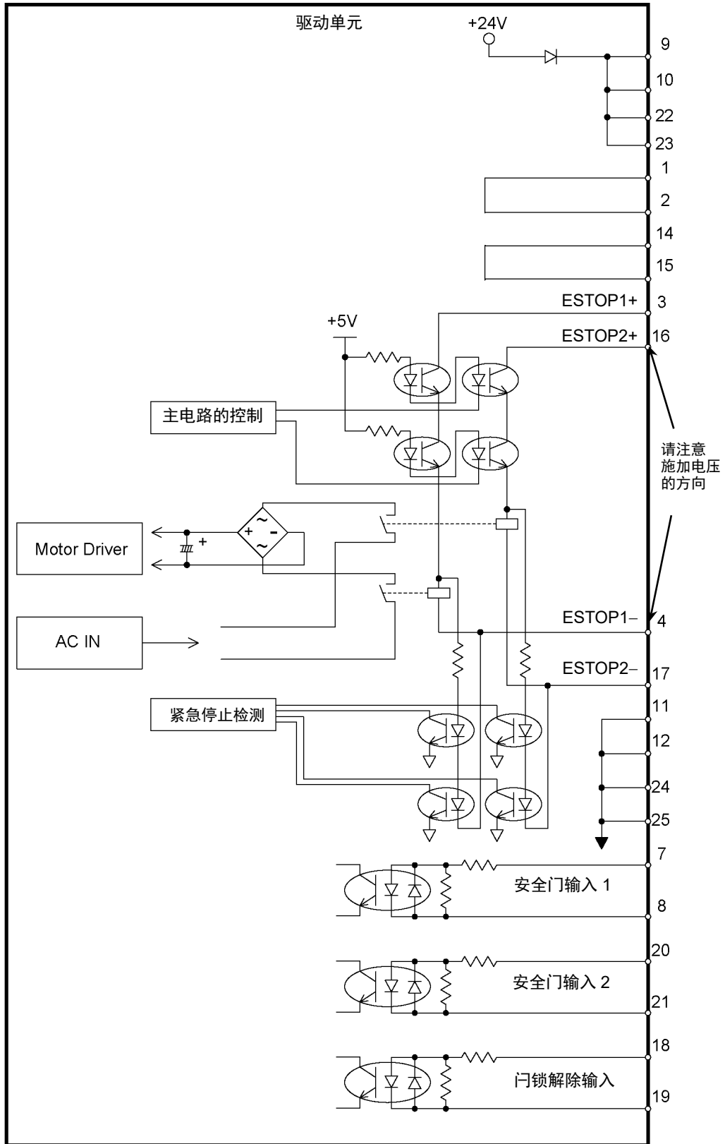
电路图
