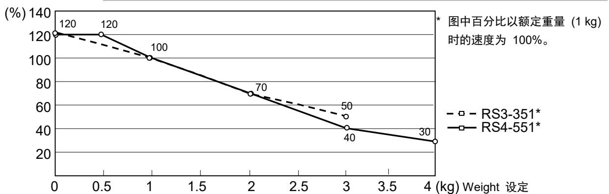
利用Weight自动设定加减速度
