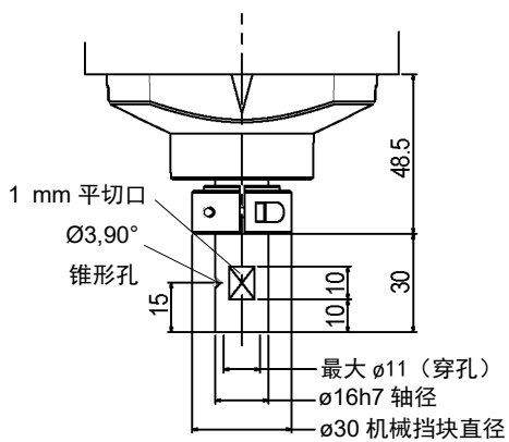
A 详图 (第 3 和第 4 关节的原点位置)
