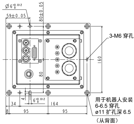
参考穿孔 (底座顶视图)
