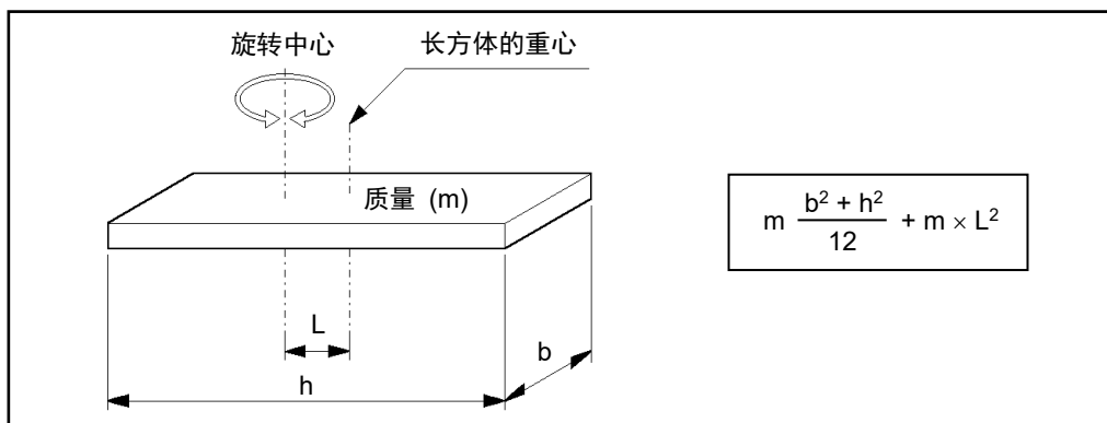
(a) 长方体的惯性力矩
