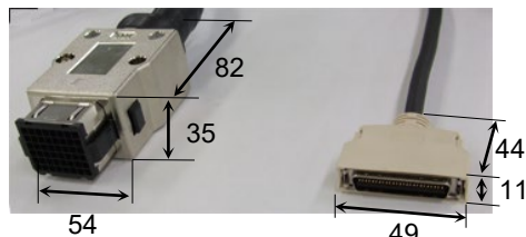
电源电缆连接器 (直型)
