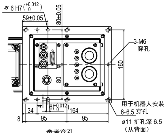
参考穿孔 (底座顶视图)
