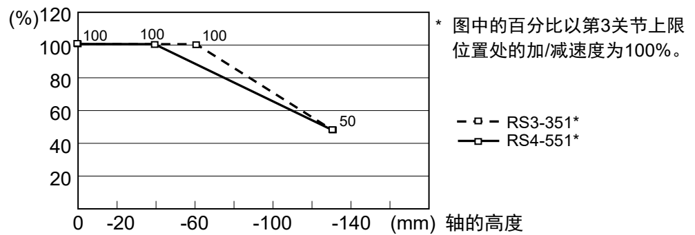
第3关节位置处的自动加减速
