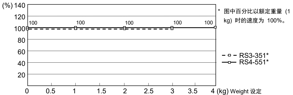
利用Weight自动设定速度
