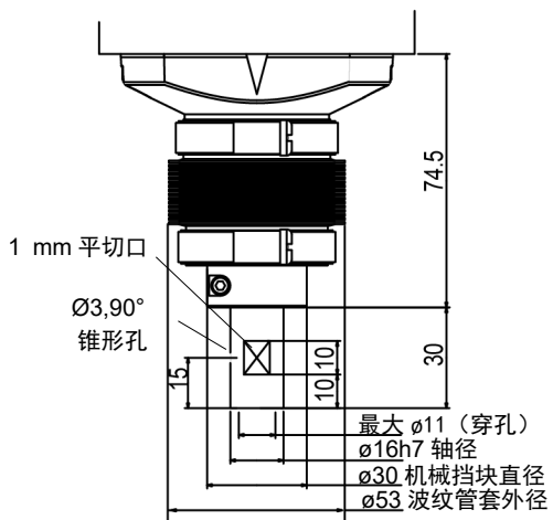
A 详图 (第 3 和第 4 关节的原点位置)
