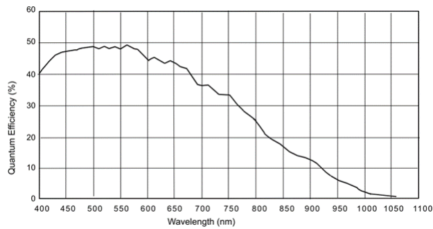
acA1600-60gm光谱灵敏度 (来自传感器数据表)
