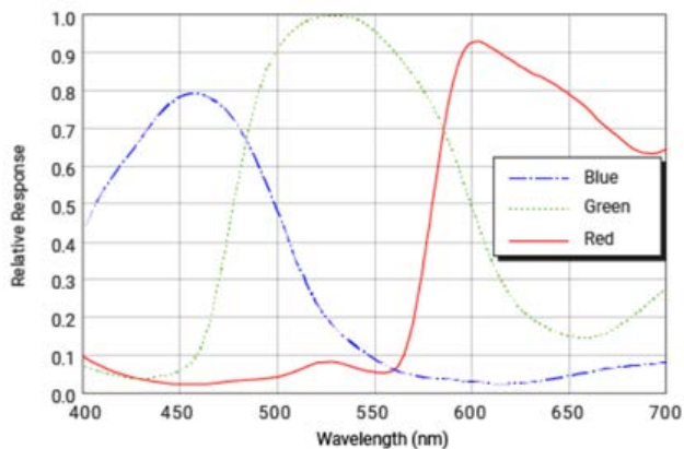
acA5472-5gc 光谱灵敏度 (来自传感器数据表)
