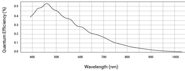
acA3800-10gm光谱灵敏度 (来自传感器数据表)
