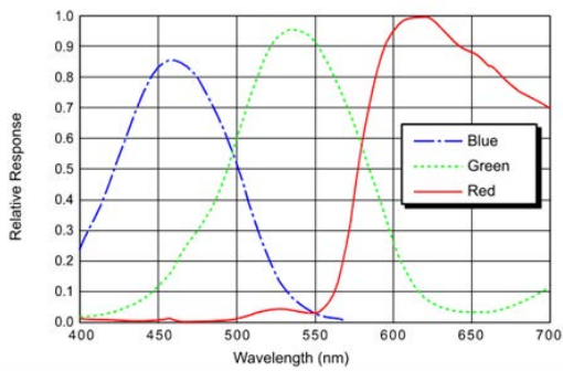
acA1600-20gc光谱灵敏度 (来自传感器数据表)
