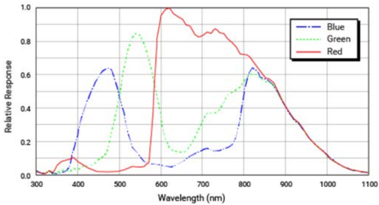
acA3800-10gc 光谱灵敏度 (来自传感器数据表)
