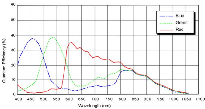
acA1600-60gc光谱灵敏度 (来自传感器数据表)
