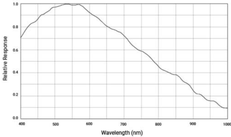
acA5472-5gm 光谱灵敏度 (来自传感器数据表)
