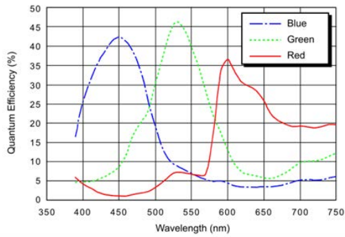
acA2500-14gc 光谱灵敏度 (来自传感器数据表)
