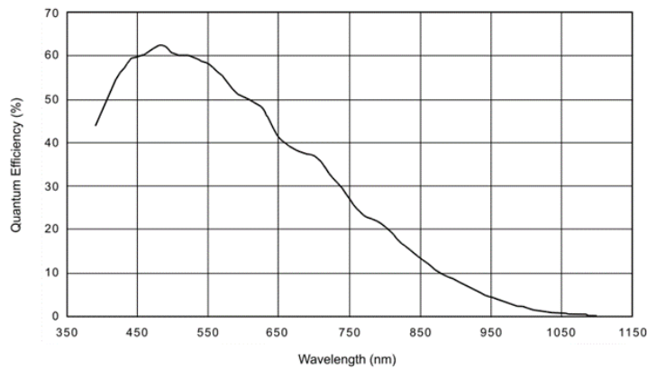
acA2500-14gm光谱灵敏度 (来自传感器数据表)
