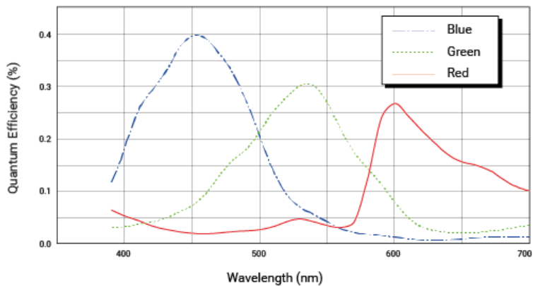
acA3800-10gc 光谱灵敏度 (来自传感器数据表)
