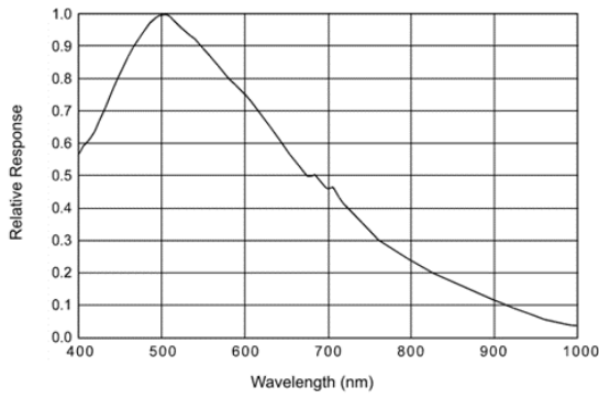
acA1600-20gm光谱灵敏度 (来自传感器数据表)
