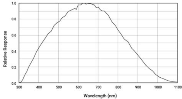
acA2500-20gm光谱灵敏度 (来自传感器数据表)
