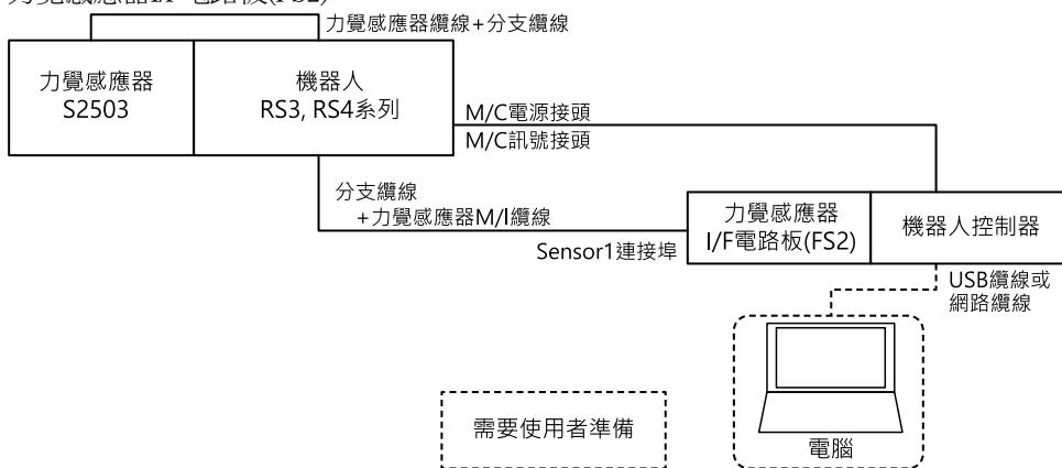
力覺感應器I/F電路板(FS2)
