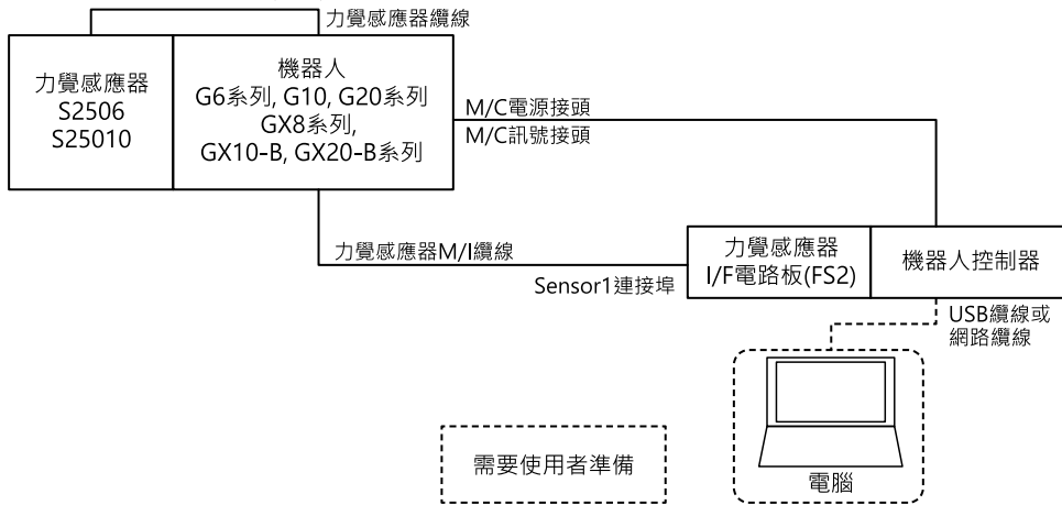
力覺感應器I/F電路板(FS2)
