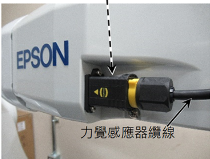
F 感應器纜線接頭
