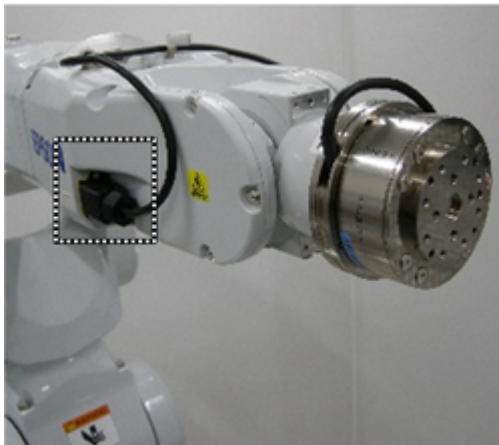
F 感應器纜線接頭
