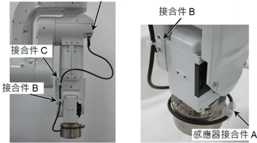
F 感應器纜線接頭
