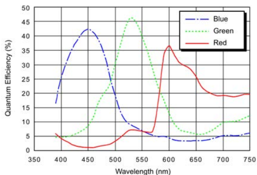
acA2500-14gc光譜響應(來自感應器資料表)
