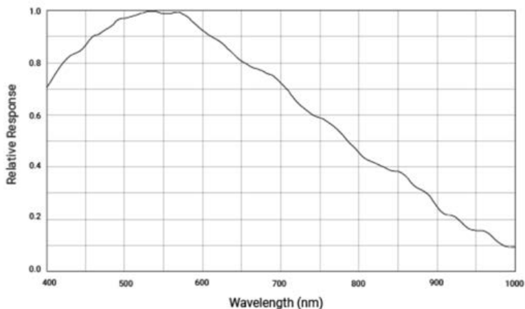
acA5472-5gm 光譜響應(來自感應器資料表)
