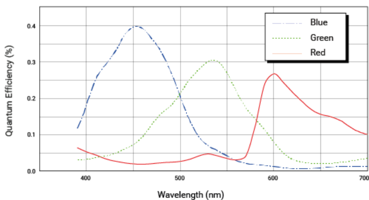
acA3800-10gc 光譜響應(來自感應器資料表)
