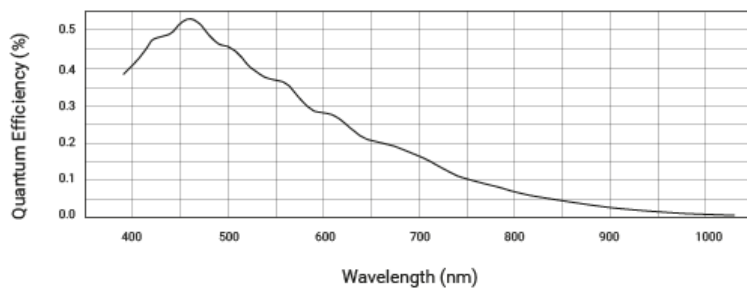
acA3800-10gm 光譜響應(來自感應器資料表)
