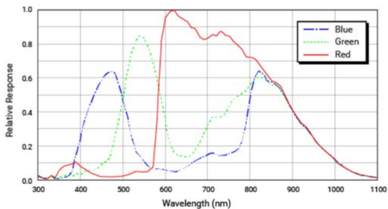
acA2500-20gc 光譜響應(來自感應器資料表)
