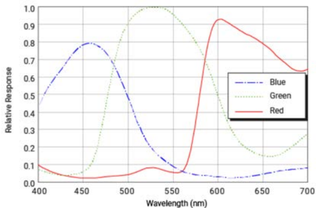
acA5472-5gc 光譜響應(來自感應器資料表)
