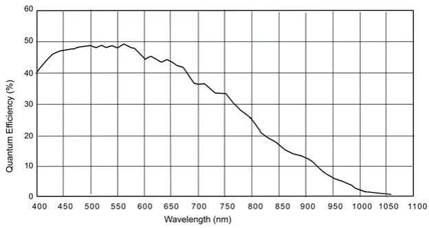
acA1600-60gm 光譜響應(來自感應器資料表)
