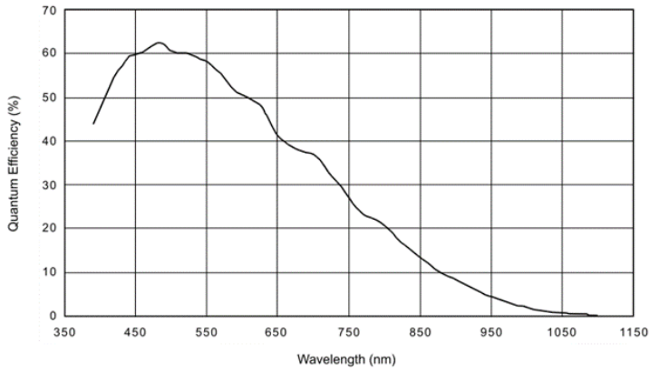
acA2500-14gm 光譜響應(來自感應器資料表)
