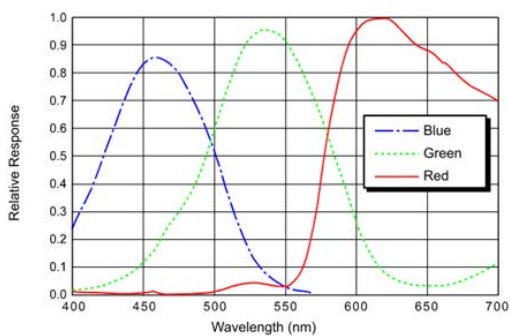
acA1600-20gc光譜響應(來自感應器資料表)
