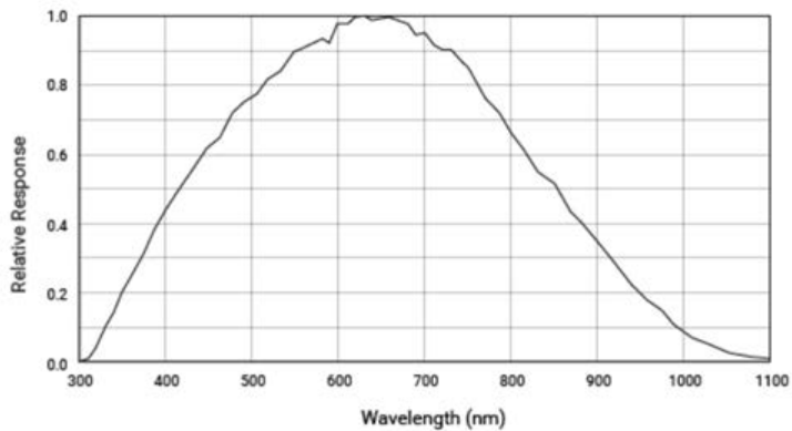
acA2500-20gm 光譜響應(來自感應器資料表)
