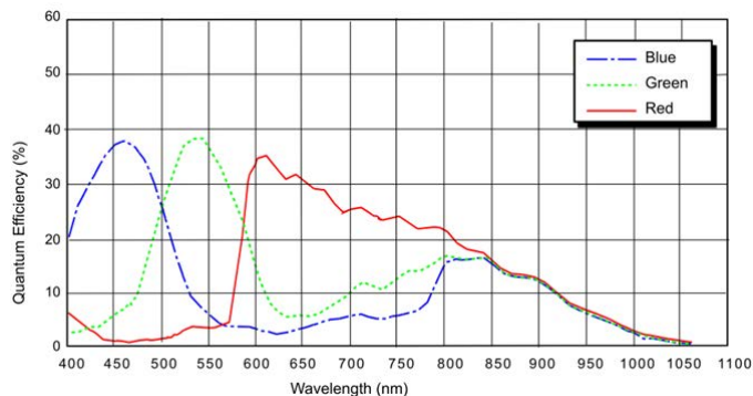
acA1600-60gc光譜響應(來自感應器資料表)
